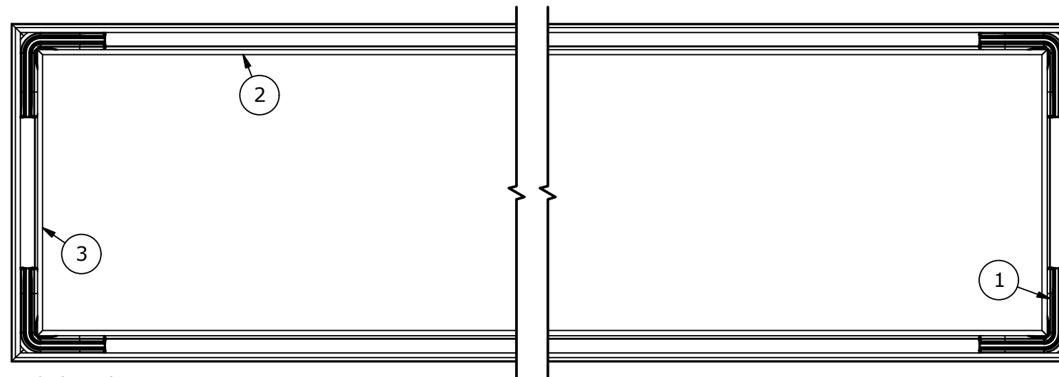
Untersicht ( 1 : 1 )
