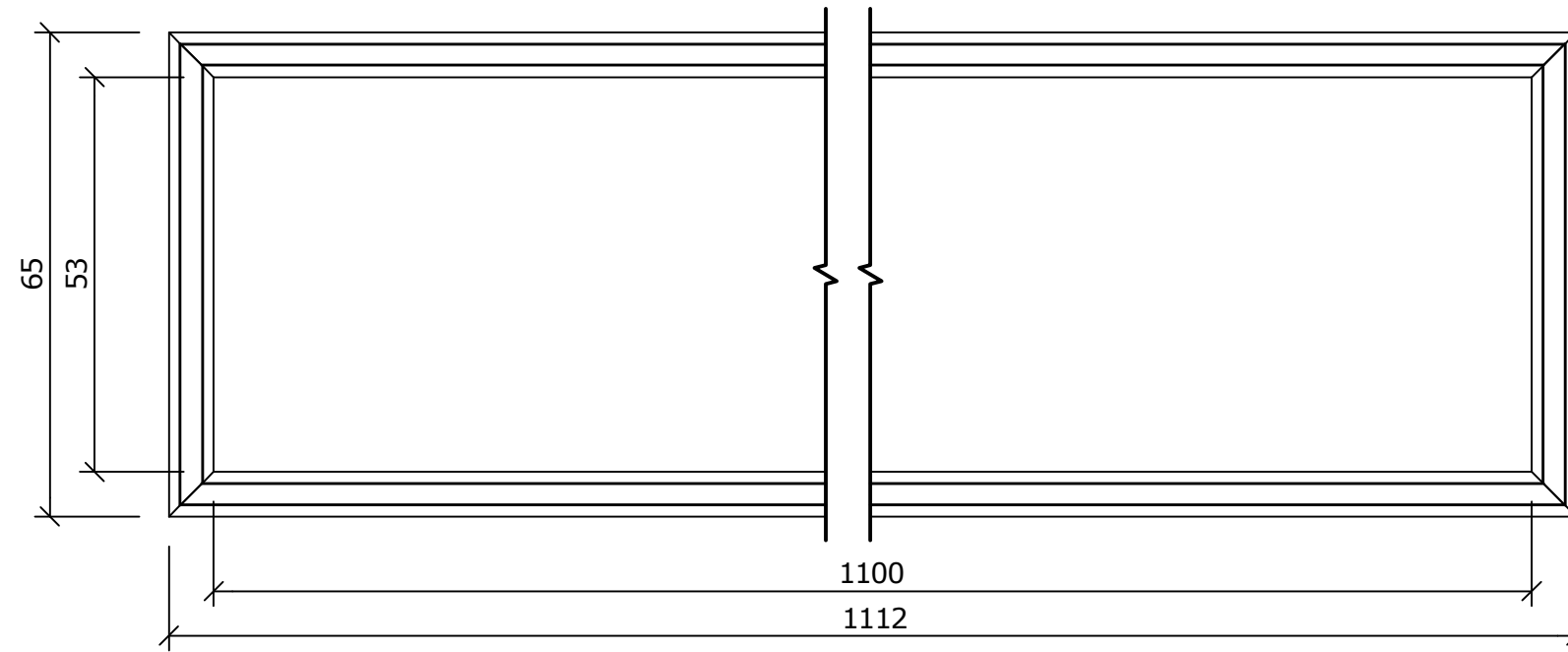
Draufsicht ( 1 : 1 )
